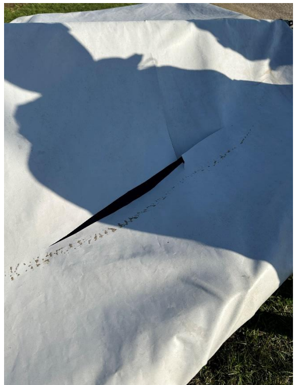
Figur 18: Presenning ødelagt i bagbord side.
